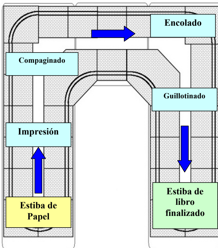
Diagrama 1. Layout de producción en "U".
